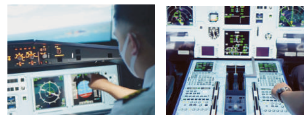
飞行模拟器 1:1 模拟驾驶舱内设有主仪表版、飞行控制组件 (FCU)，以及多用途控制及显示组件 (MCDU)
